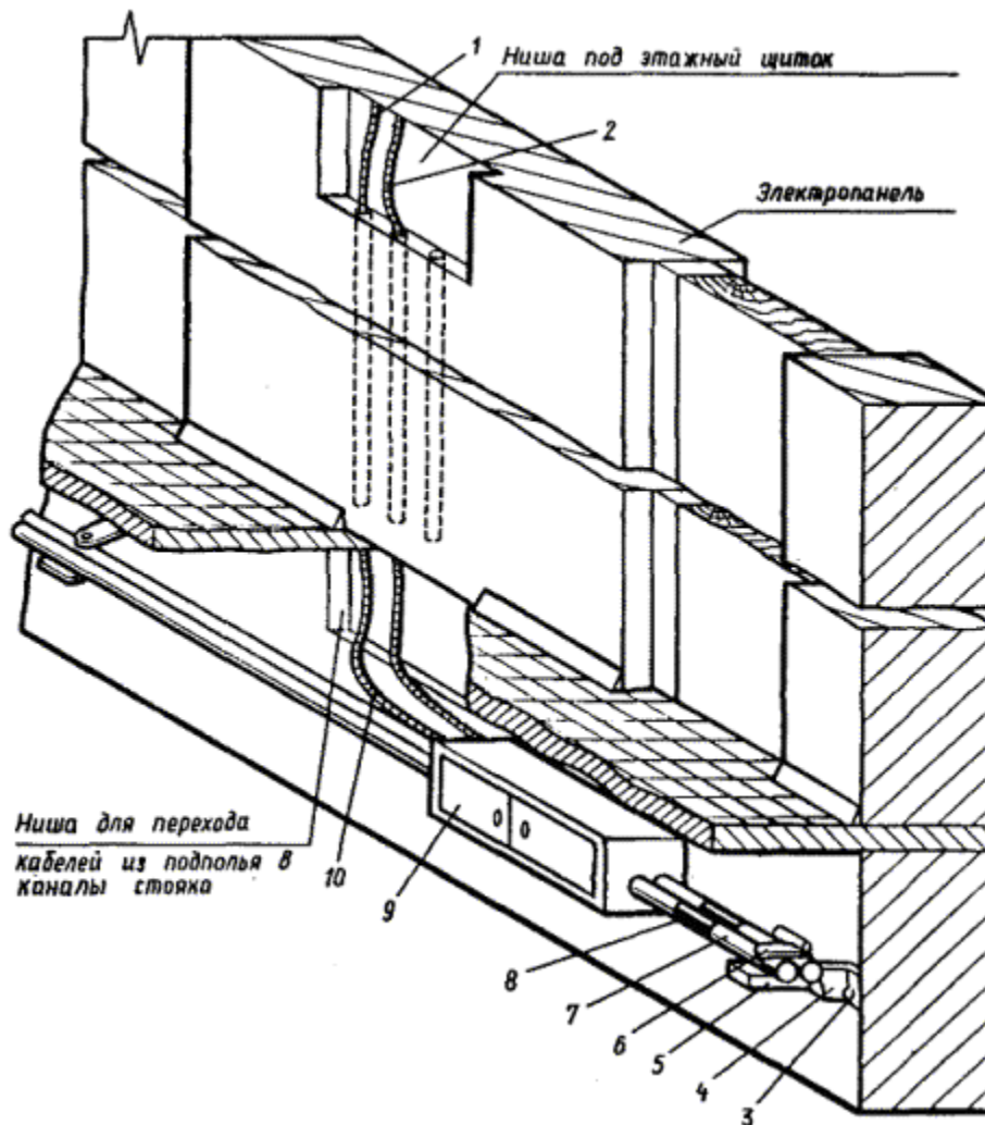
Рис. 6.6. Пример прокладки кабелей по подполью в виниловых трубах и металлорукавах:
