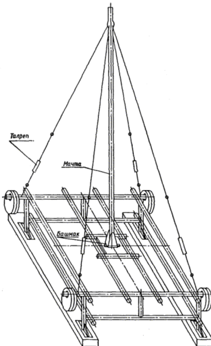
Рис. 4.3. Передвижная конструкция крепления мачты
