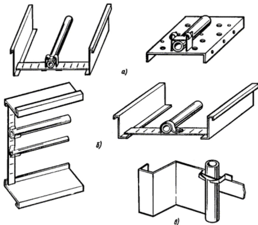
Рис. 6.2. Примеры крепления проложенного в лотках кабеля:
