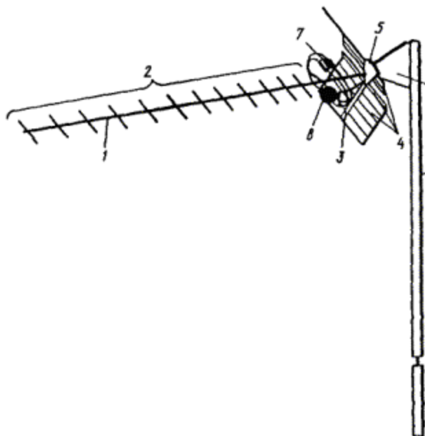
Рис. 4.4. Общий вид антенны АТКГ (В) - 5.1.21-41.0:
