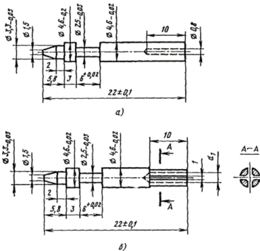
Рис. 2.2. Центральная втулка разъема. Материал - латунь:
