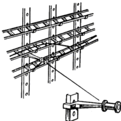
Рис. 6.1. Пример прокладки кабеля на лотках по раскатным роликам
