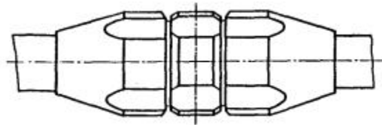
Рис. 6.9. Конструкция соединителя СКП 2,7/28,6 и его основные размеры
