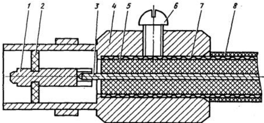
Рис. 2.4. Соединение кабеля с разъемом.
