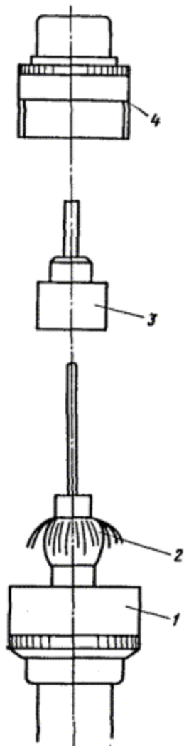
Рис. 8.1. Монтаж разъемов, входящих в комплект ГС производства ВНР. Длина разделки кабеля равна длине монтируемого разъема плюс 10 мм.
