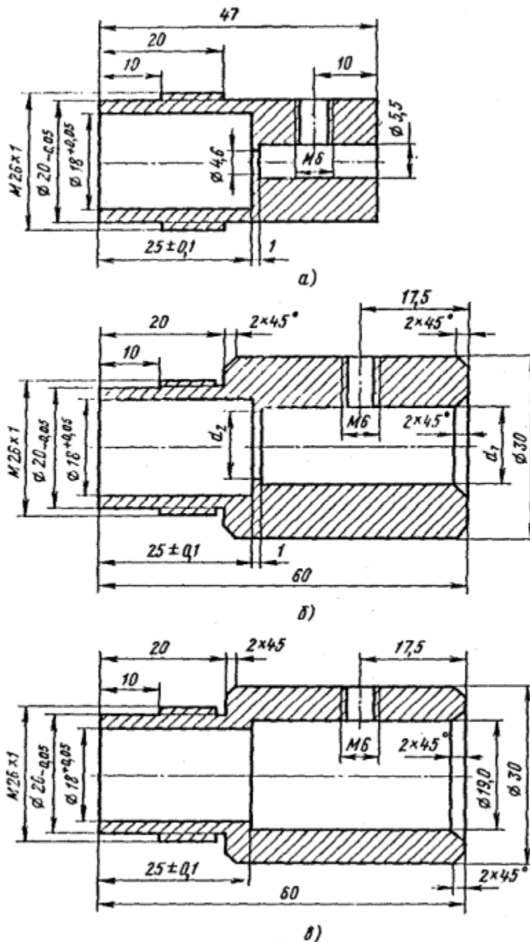
Рис. 2.1. Корпус разъема. Материал - латунь:
