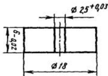
Рис. 2.3. Шайба. Материал - фторопласт-4 или полиэтилен
