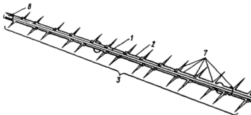
Рис. 4.5. Общий вид логопериодической антенны IV, V ТВ диапазонов:
