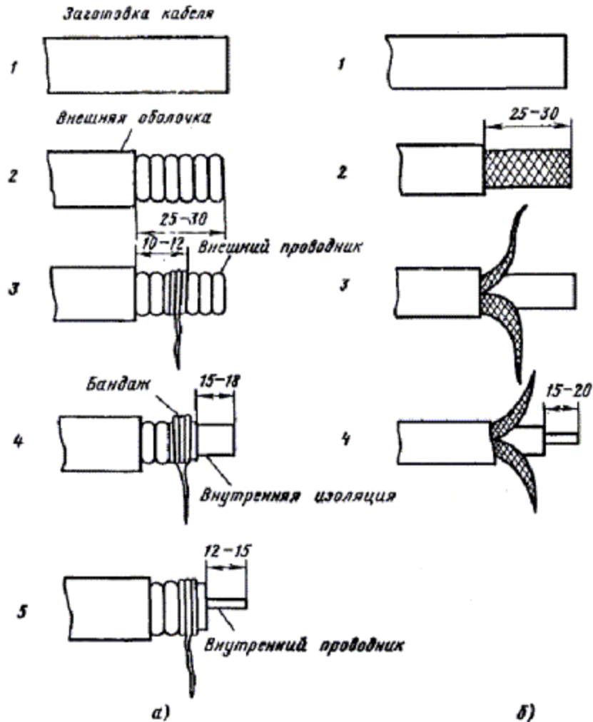
Рис. 8.3. Последовательность операций по разделке кабелей:
