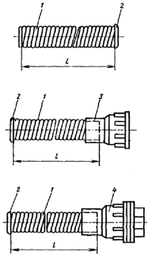
Рис. 6.5. Примеры заготовки металлорукавов для защиты кабеля:
