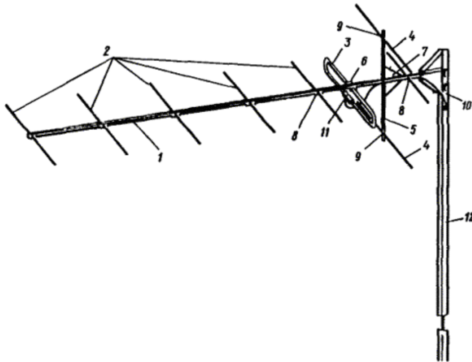
Рис. 4.2. Общий вид канальной антенны повышенной помехозащищенности III ТВ диапазона:
