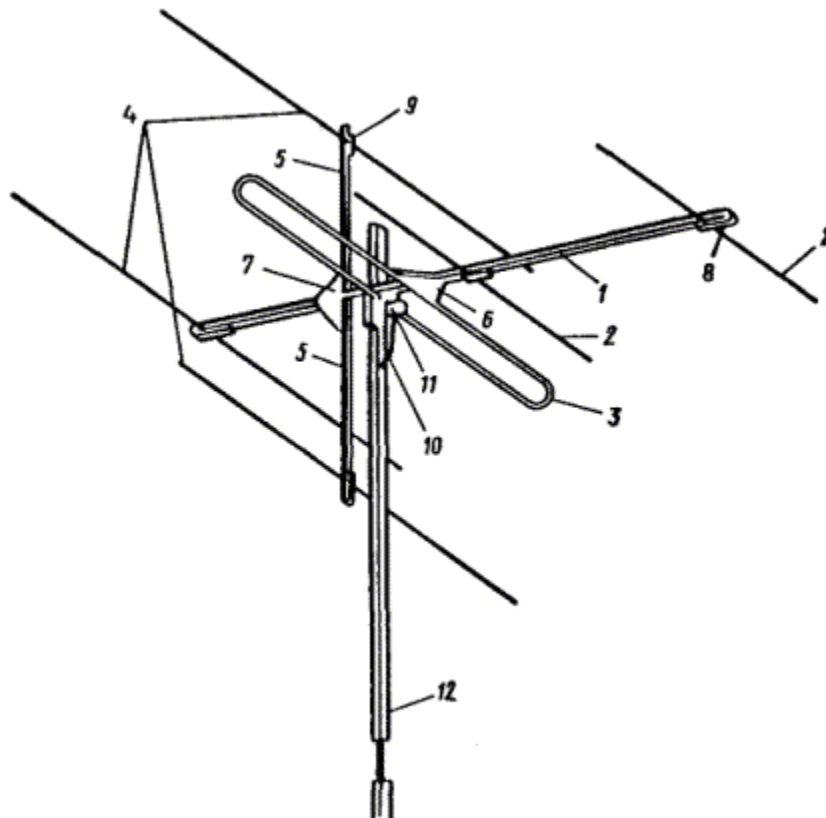
Рис. 4.1. Общий вид канальной антенны повышенной помехозащищенности I, II ТВ диапазонов:
