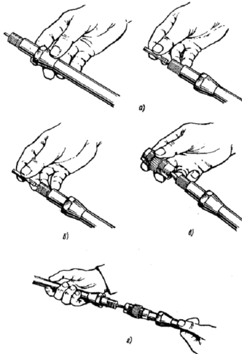
Рис. 6.10. Монтаж соединителя типа СКП
