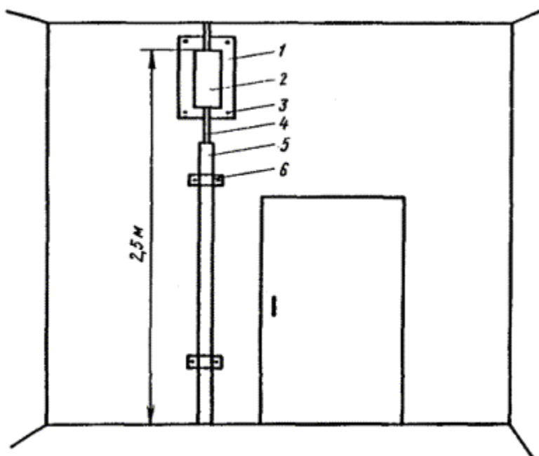
Рис. 7.1. Пример установки распределительного устройства на лестничной клетке:
