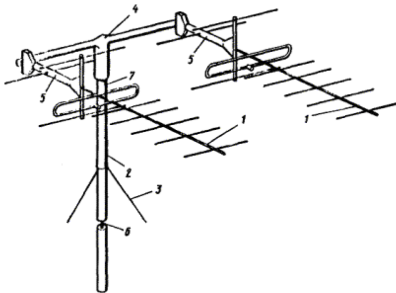
Рис. 4.7. Общий вид сдвоенной антенны крепления сдвоенной антенны на одной мачте:
