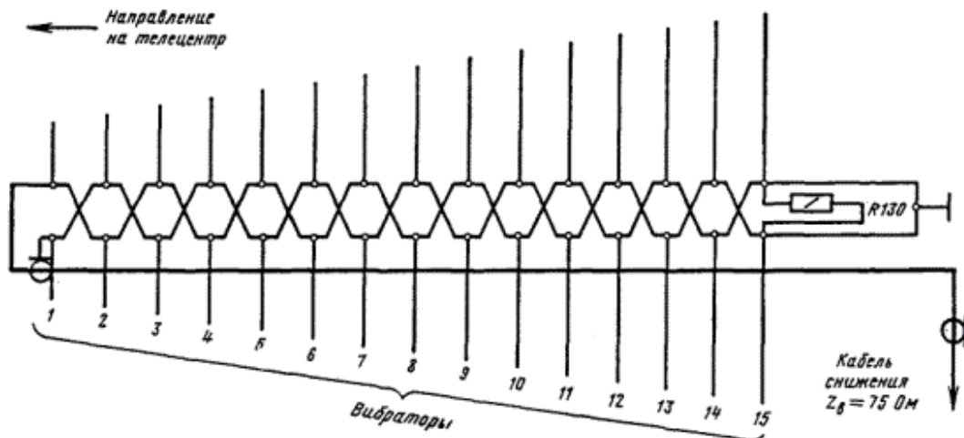
Рис. 4.6. Схема подключения вибраторов антенн IV, V ТВ диапазонов частот
