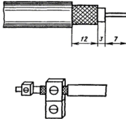
Рис. 8.2. Включение магистральных кабелей в ГС и усилителей производства ВНР:
