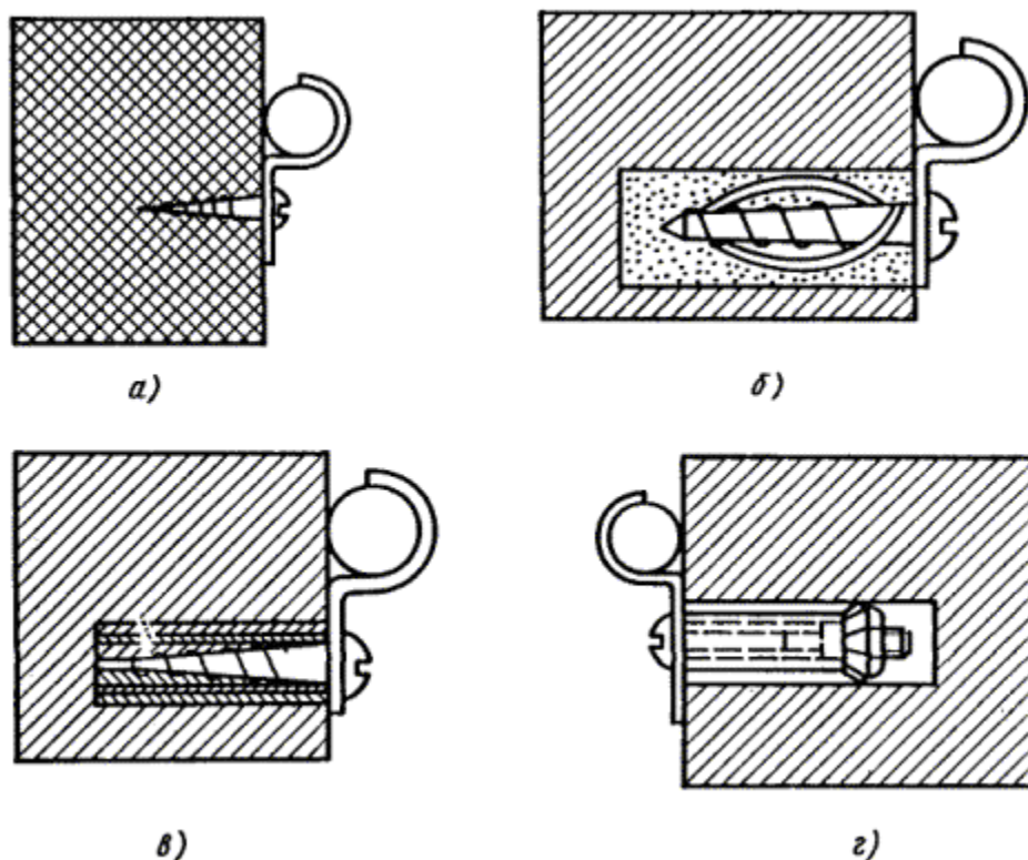
Рис. 6.7. Примеры крепления кабелей к стенам зданий:
