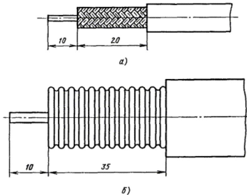
Рис. 2.5. Разделка концов кабелей для армирования разъемами:
