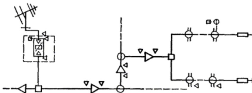
Рис. П.5. Точки измерений на распределительной сети системы
